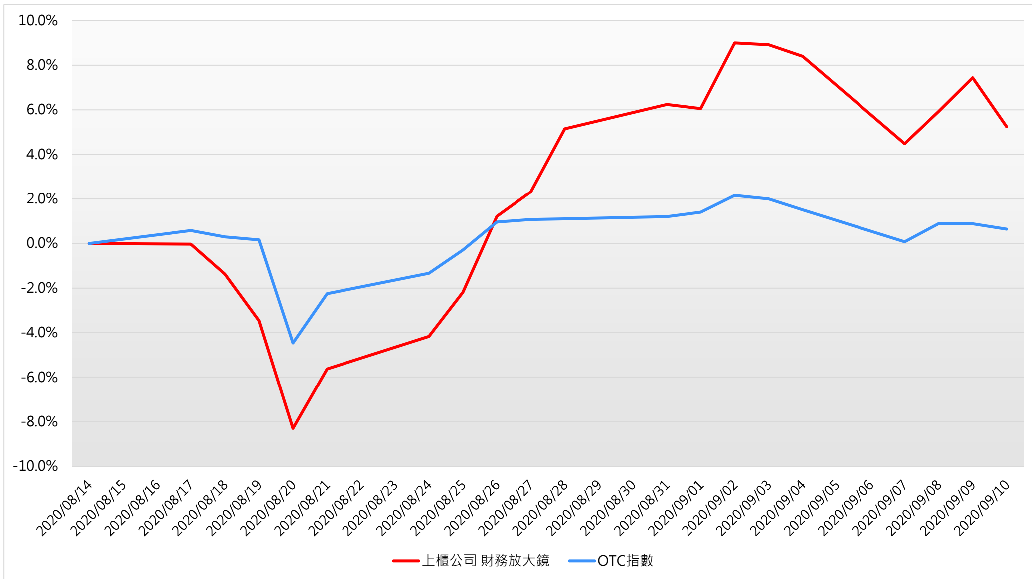
圖5.「上櫃公司 財務放大鏡」投資組合績效
