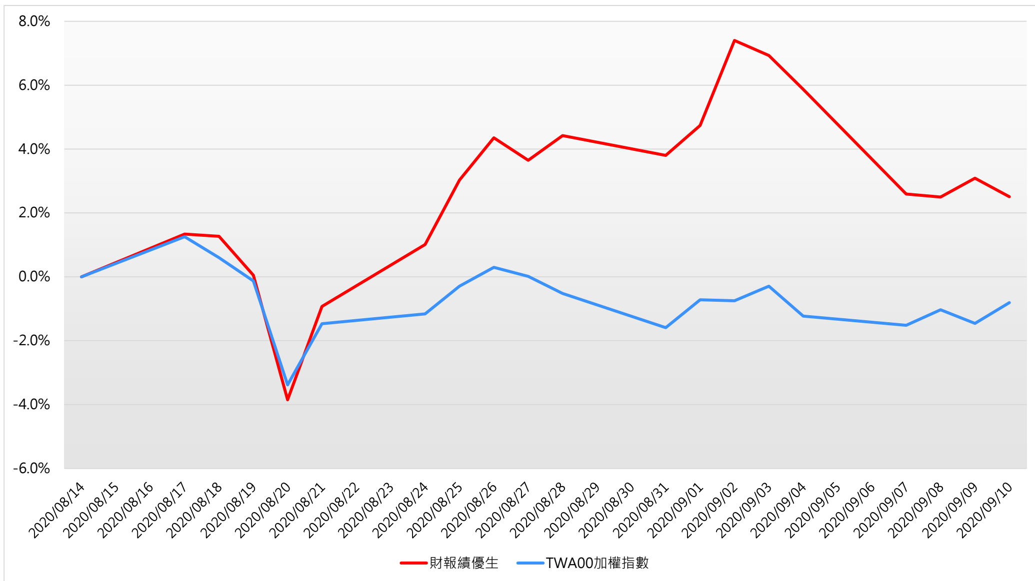
圖2.「財報績優生」投資組合績效
