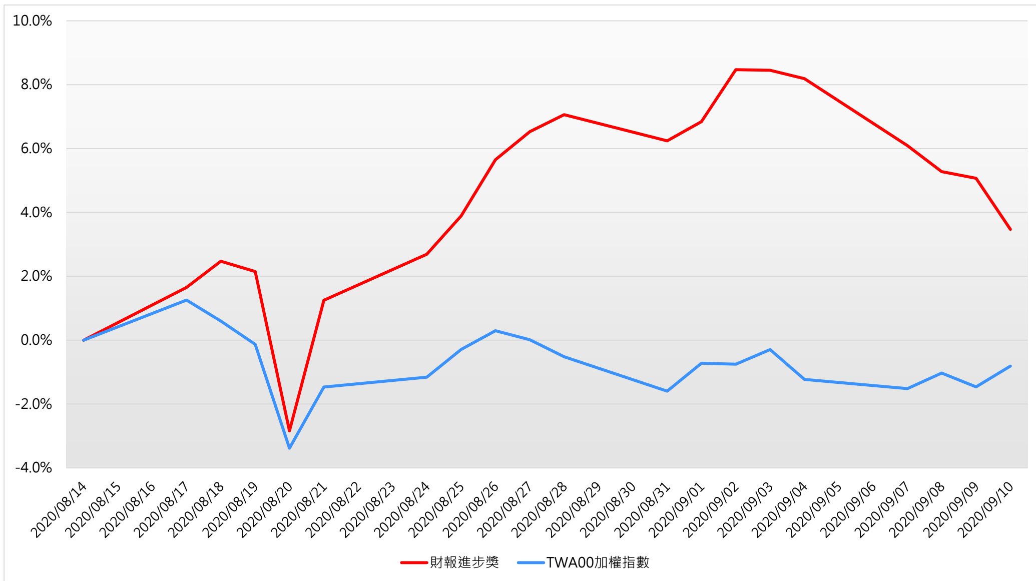
圖3.「財報進步獎」投資組合績效
