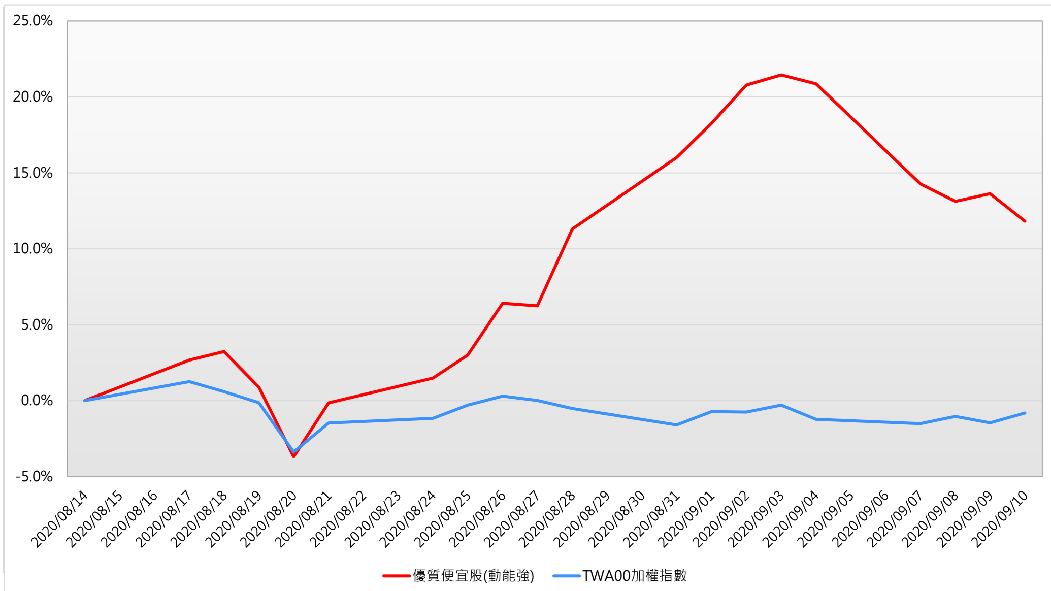
圖1.「優質便宜股(動能強)」投資組合績效
